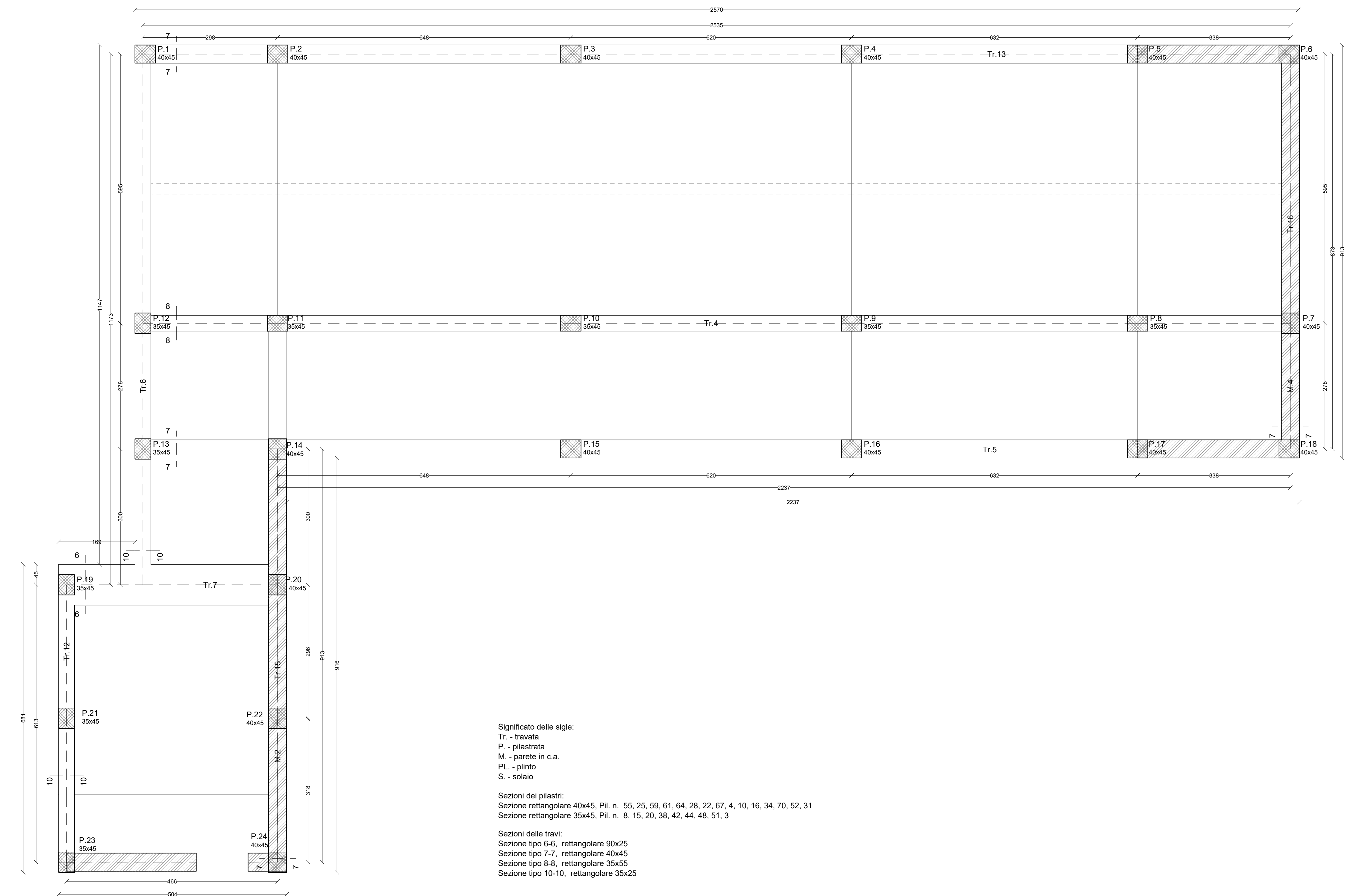
Impalcato a quota +160.0
